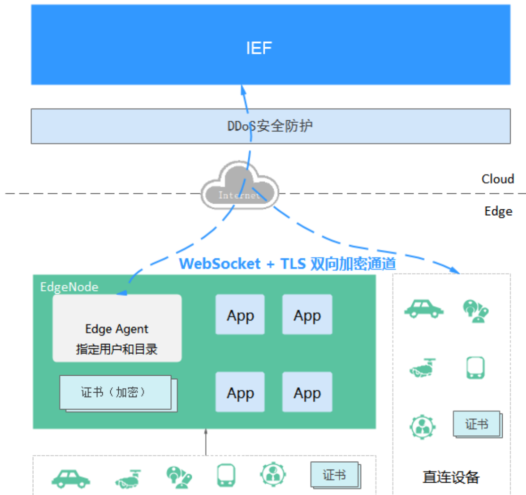
图 3-4 IEF 安全性方案
